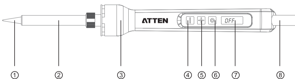
图1-1 (产品主视图)
