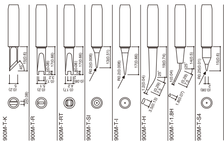
烙铁嘴规格图（900M系列）
